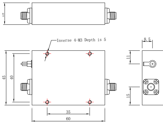
UNIT: mm XB-07A
